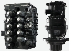
MCV와 선회모터
